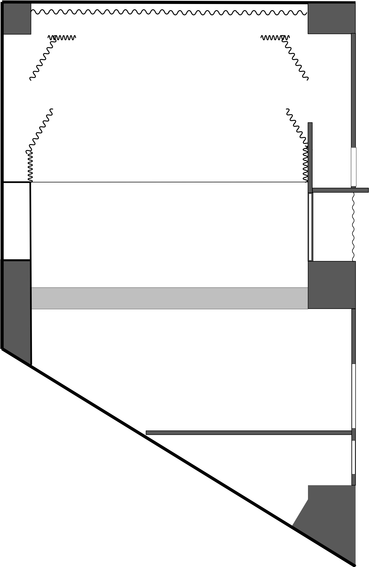
平面白図①袖幕吊り込み例(2016.06.01修正版) 元図 A4 1/50 (割幕は開ききりで間口4.3m)
