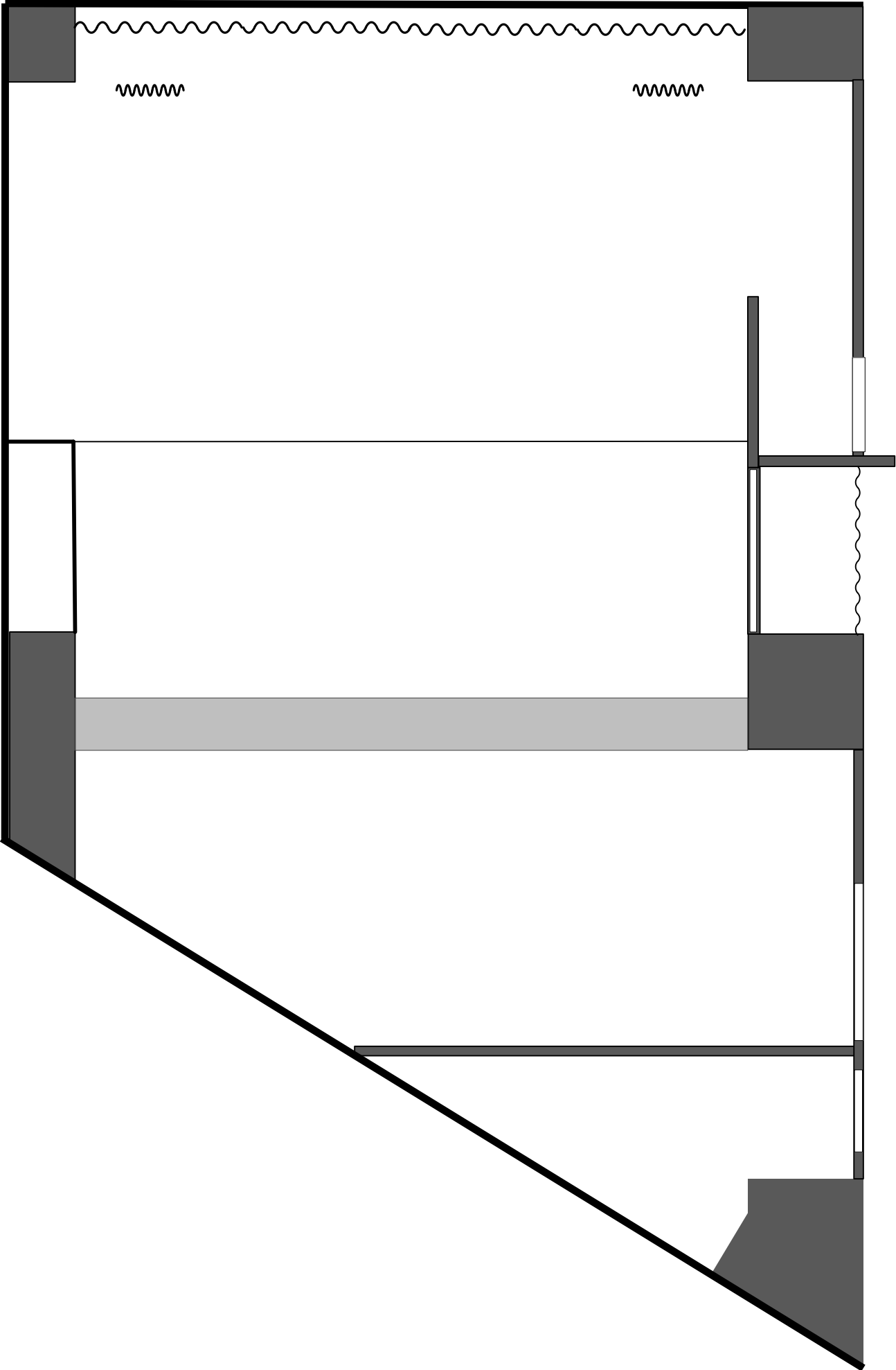
平面白図②袖幕なし(2016.06.01修正版) 元図 A4 1/50 (割幕は開ききりで間口4.3m)
