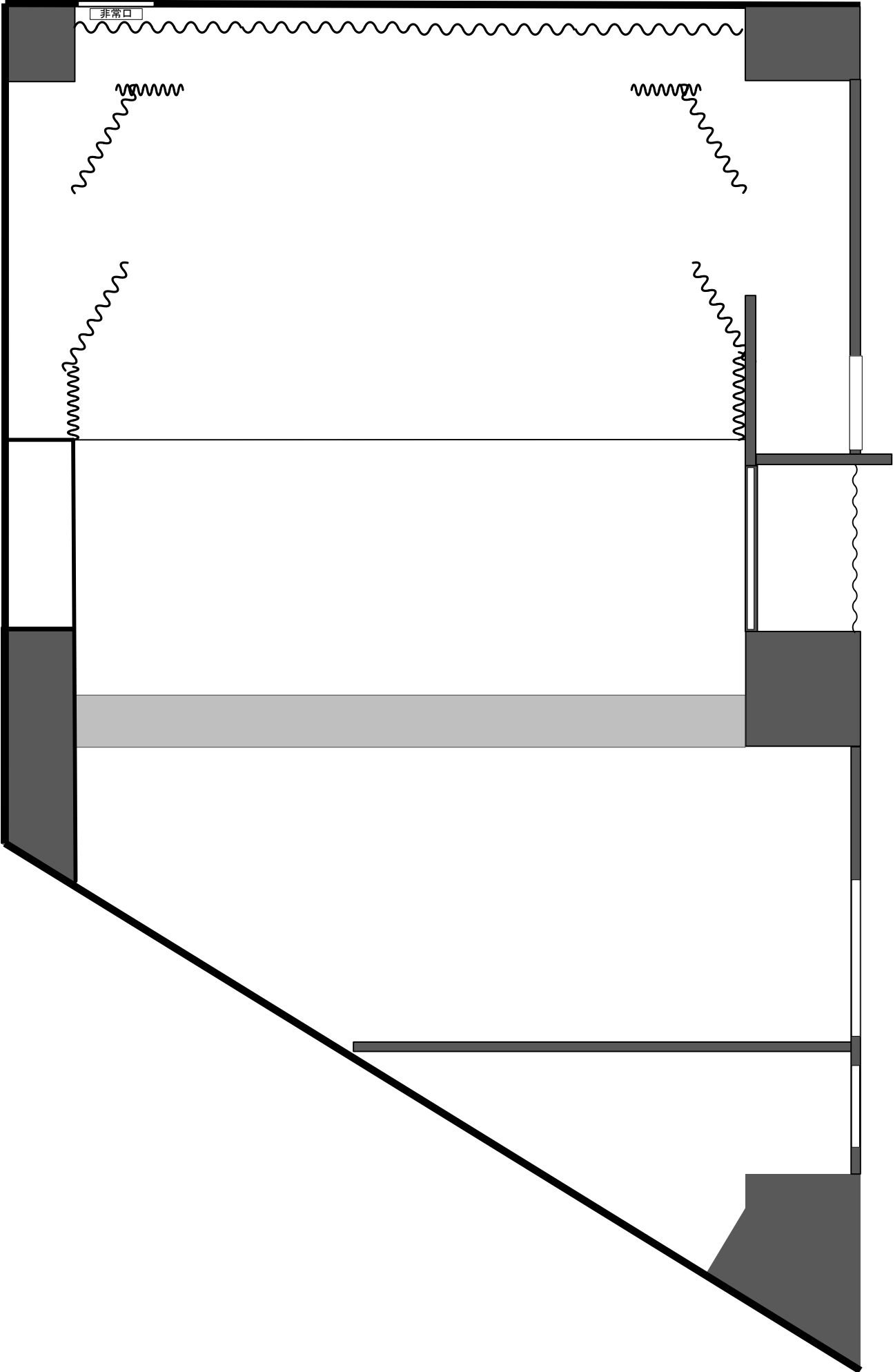
平面白図①袖幕吊り込み例(2018.12.20修正版) 元図 A4 1/50 (割幕は開ききりで間口4.3m)
