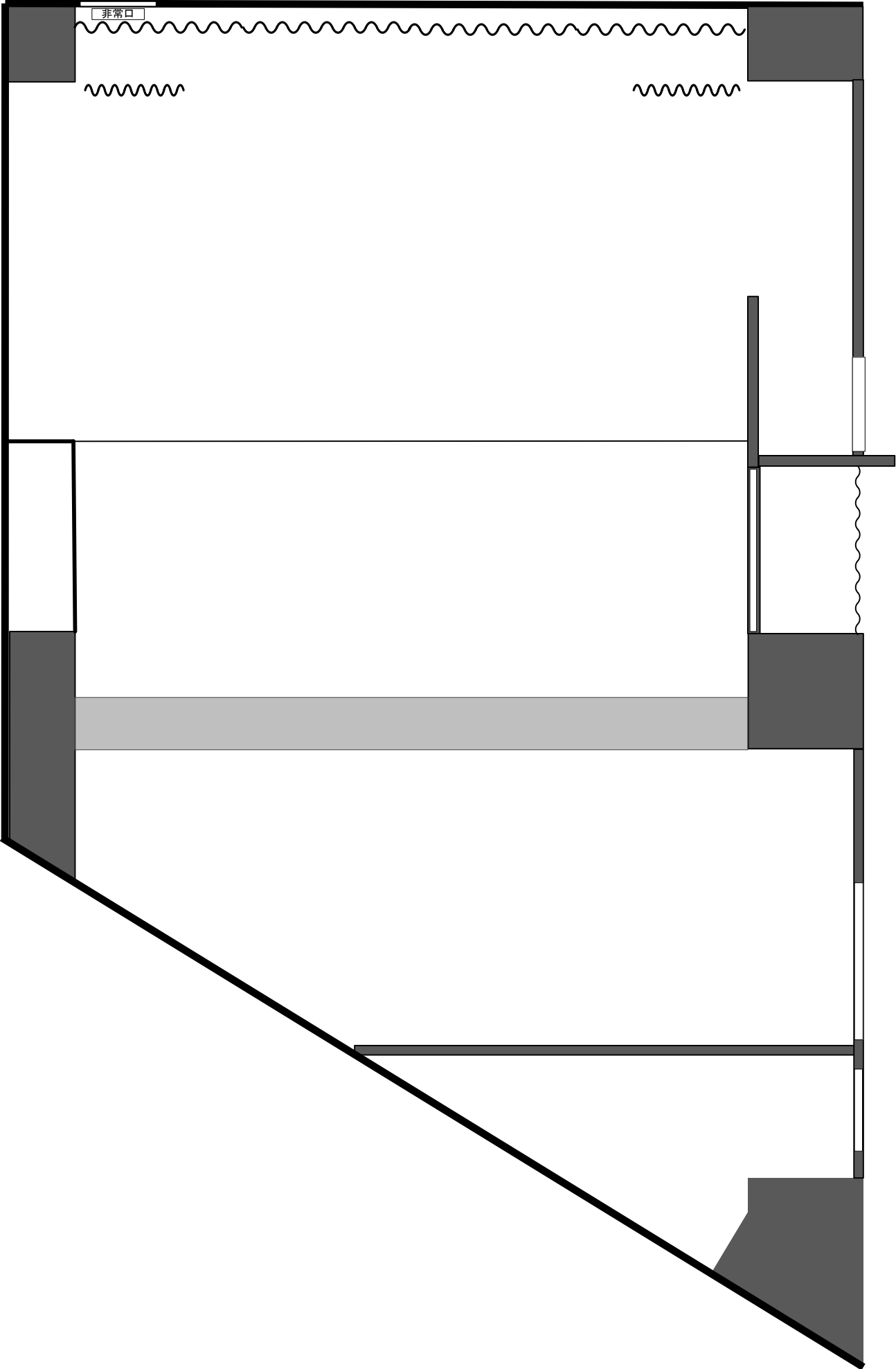
平面白図(2019.05.15修正版) 元図 A4 1/50 (割幕は開ききりで間口4.3m)
